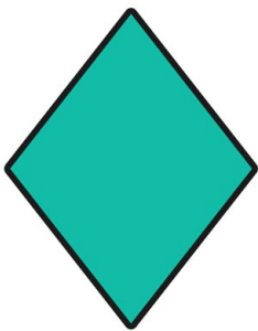
rhombus
