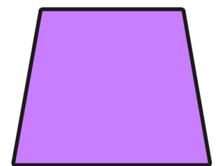
trapezium
